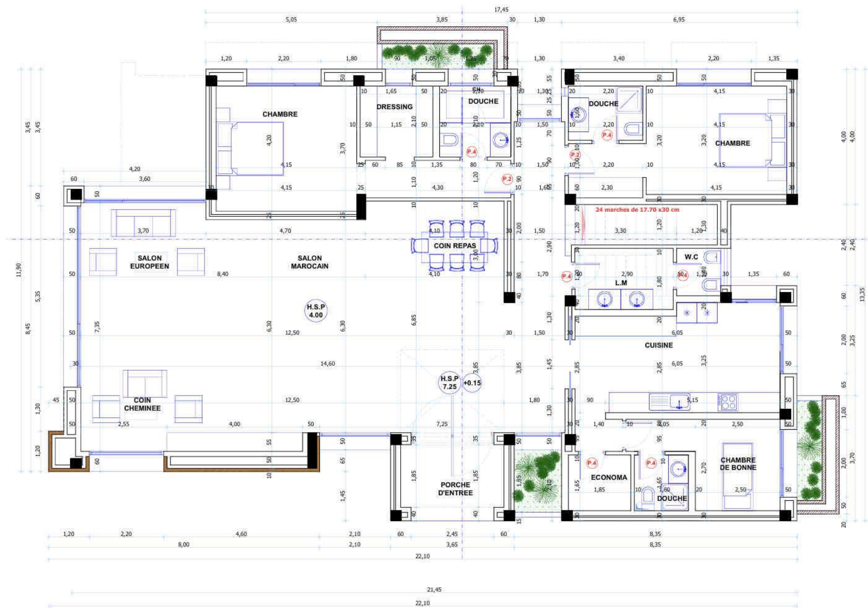
PLAN RDC
